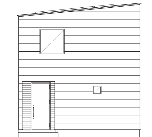
北側立面図
