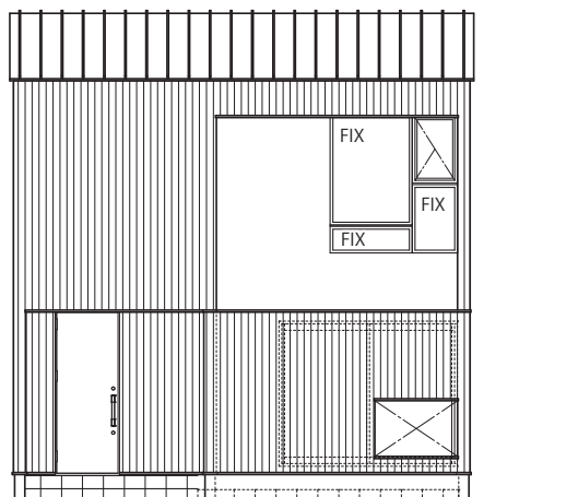
西側立面図
