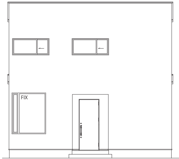
西側立面図
