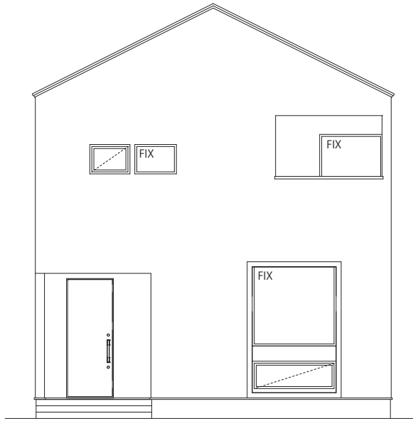
南側立面図
